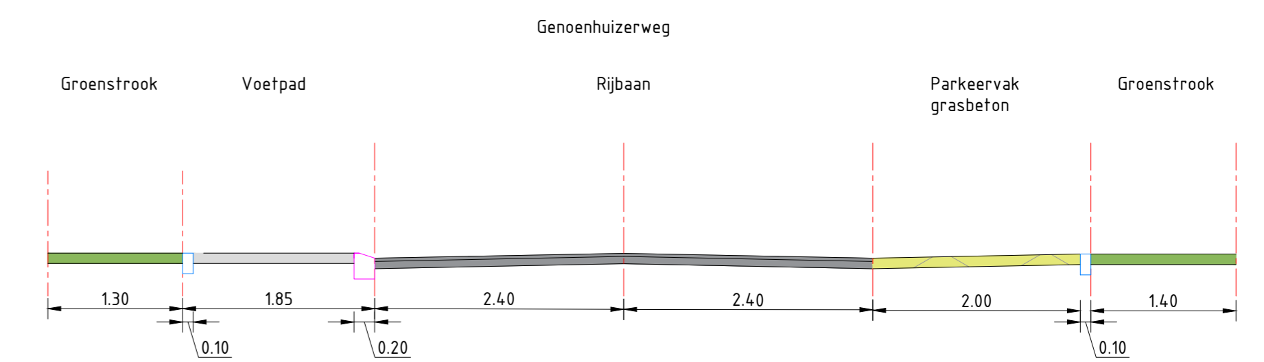
Principe doorsnede A-A Schaal 1:50
